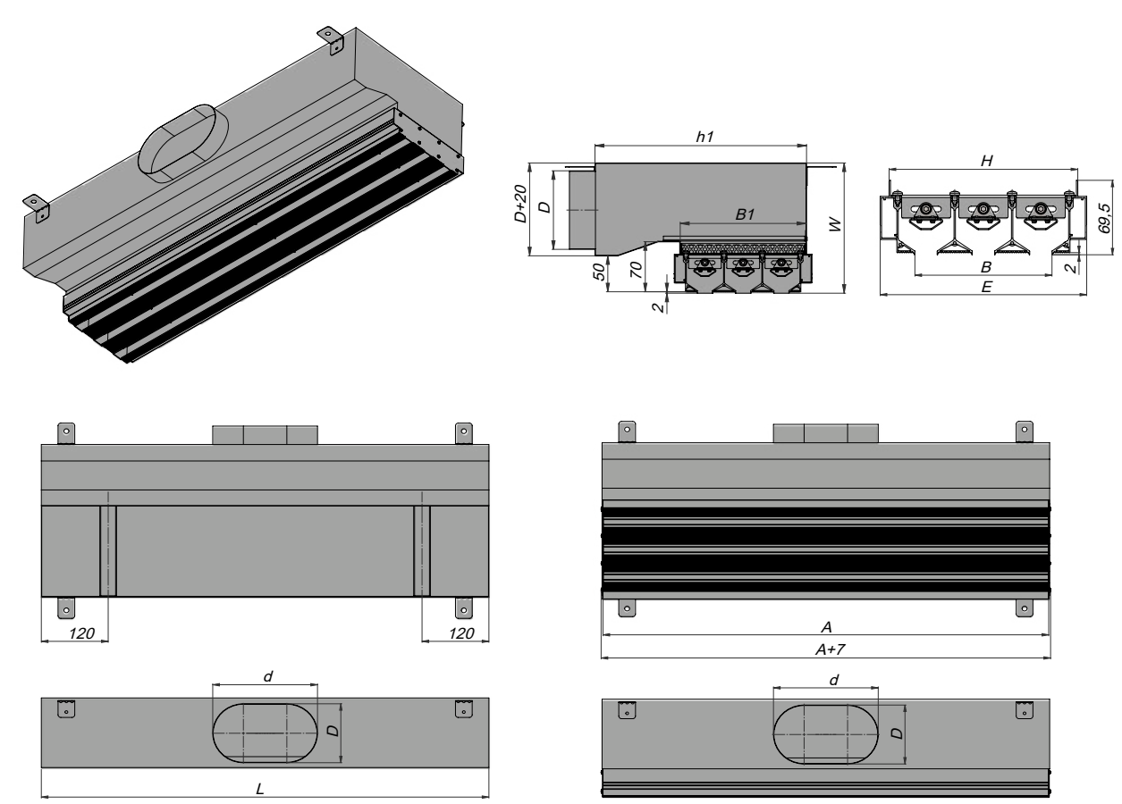
Габаритно-посадочные размеры щелевого диффузора A-Line-IN + уменьшенная КСД-U-O с овальной вырезкой А — ширина щелей, В — высота щелей
