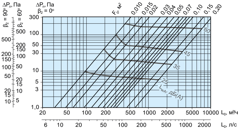
Аэродинамические и акустические характеристики решеток BETA-CI, BETA-CI-R1 при углах наклона жалюзи \alpha_1 = 0^\circ, \alpha_2 = 0^\circ
