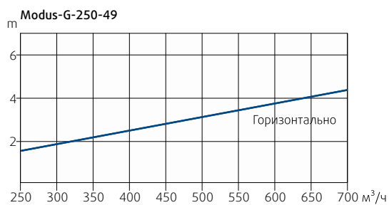
Диаграмма 18: Дальность броска изотермической струи (горизонтальная подача воздуха) при конечной скорости 0,2 м/с
