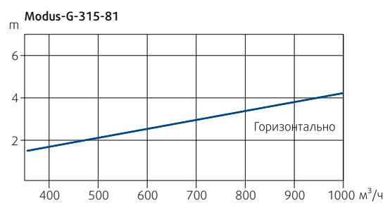
Диаграмма 20: Дальность броска изотермической струи (горизонтальная подача воздуха) при конечной скорости 0,2 м/с
