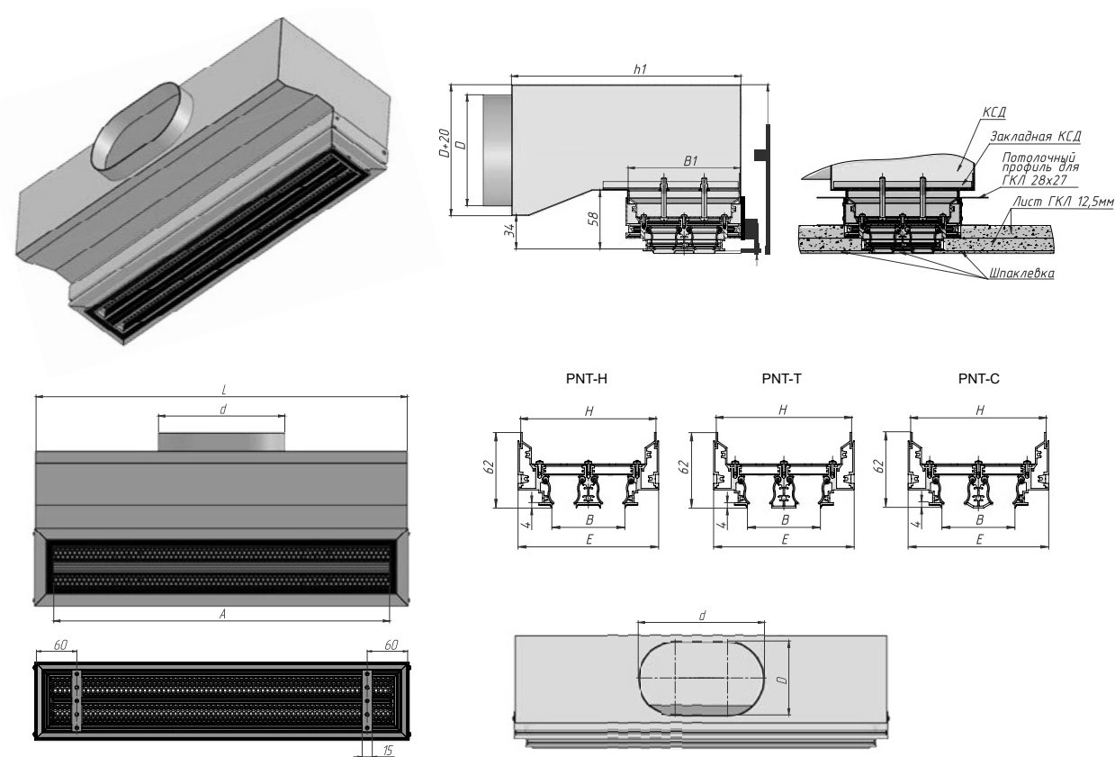
Габаритно-посадочные размеры диффузора PNT + уменьшенная РВ-PNT-0-U-0 с овальной вырезкой А — ширина щелей, В — высота щелей
