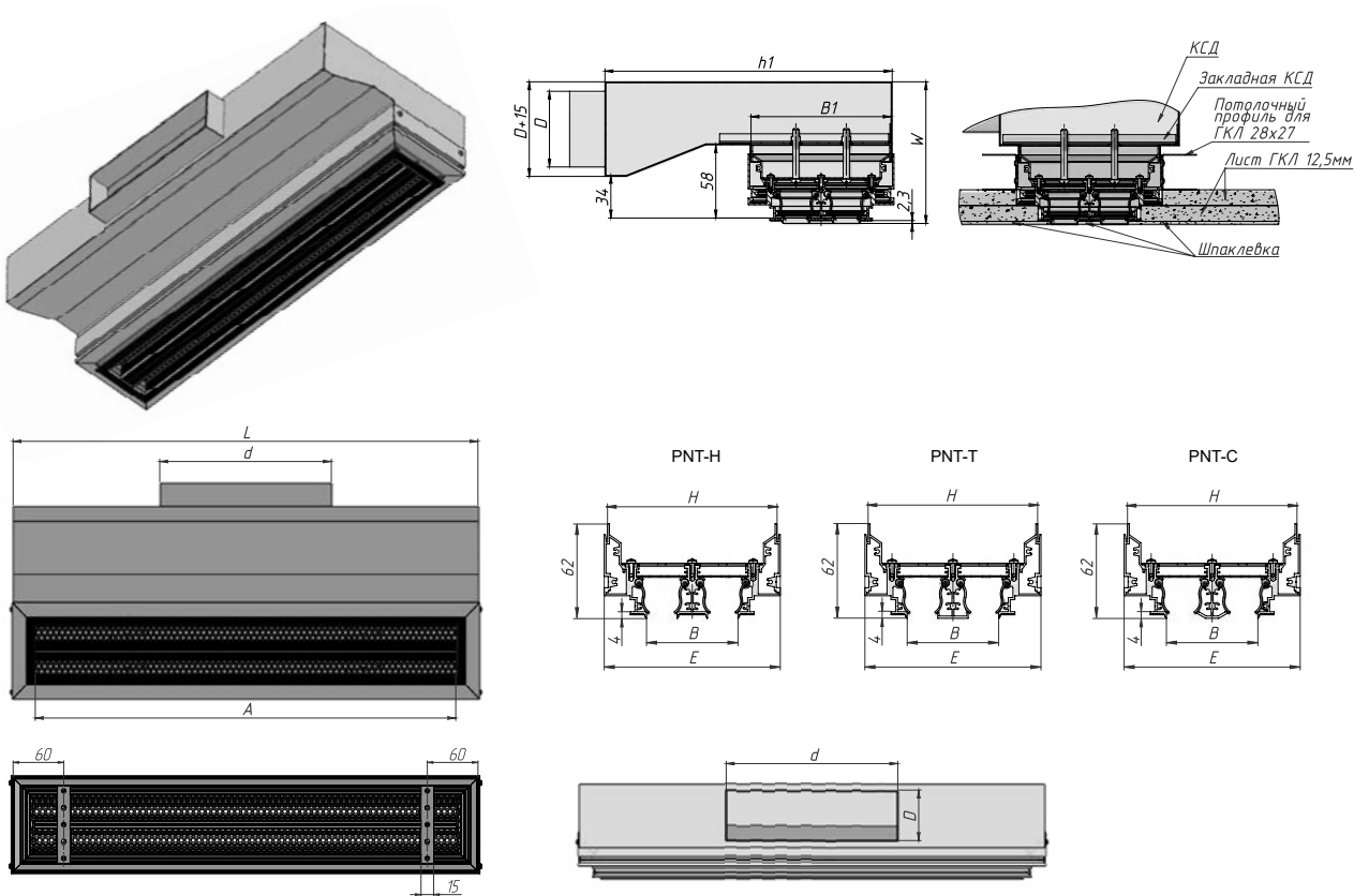
Габаритно-посадочные размеры диффузора PNT + уменьшенная РВ-PNT-0-Р с прямоугольной вырезкой А — ширина щелей, В — высота щелей
